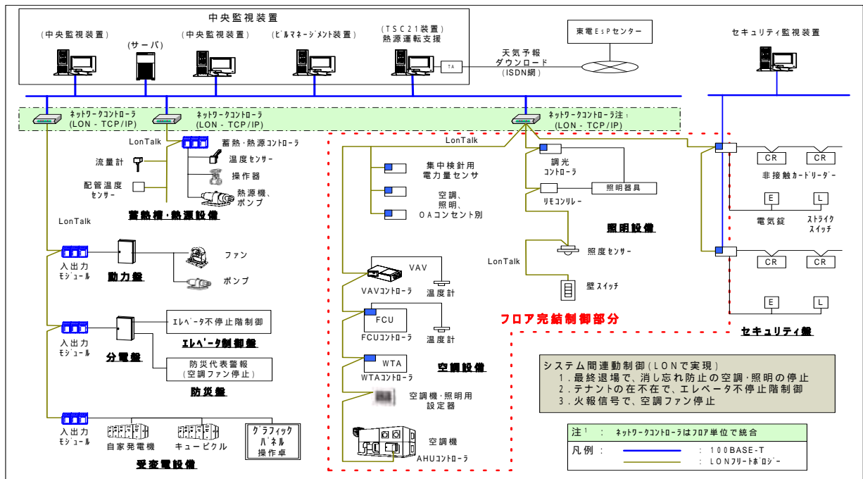
図 中央監視設備・システム構成図
